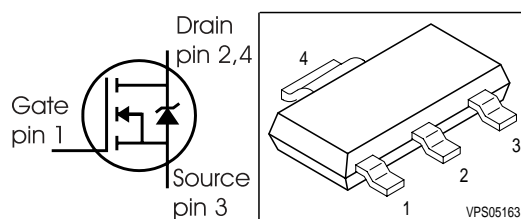
PG-SOT-223
